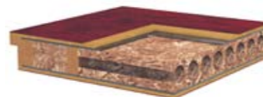
Przekrój drzwi AGAT i OPAL płyta wiórowa + blachy aluminium
